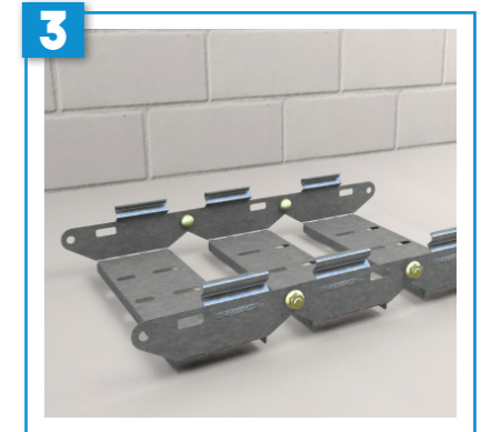
Armá la curva con la cantidad que requiera la instalación.
